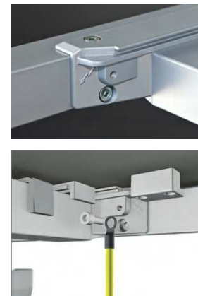
Punto de conexión a toma de tierra / Earth wire point Point de connexion de prise en terre / Anschlusspunkt für die Schutzleitung zur Erdung
